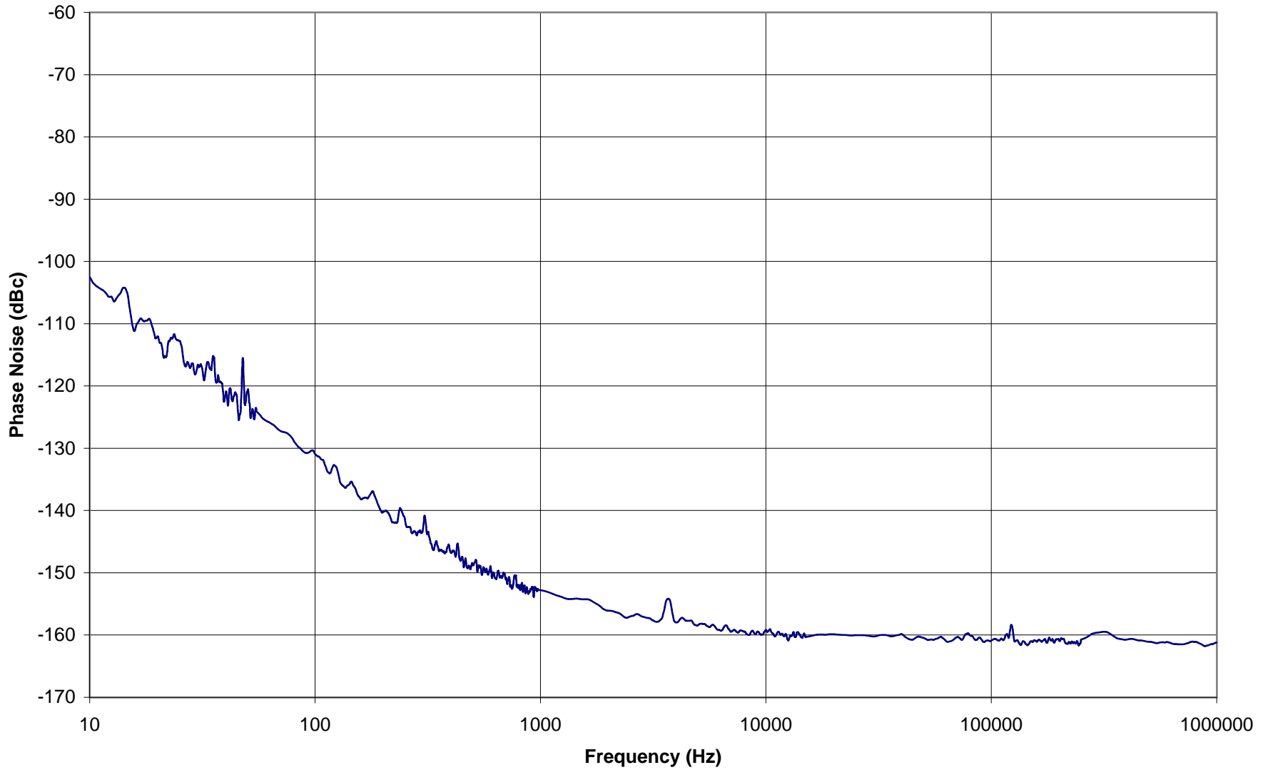
50MHz OCXO PN NXOS-0005
